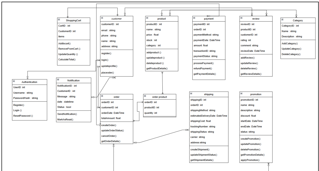
Hình 7.sơ đồ lớp
