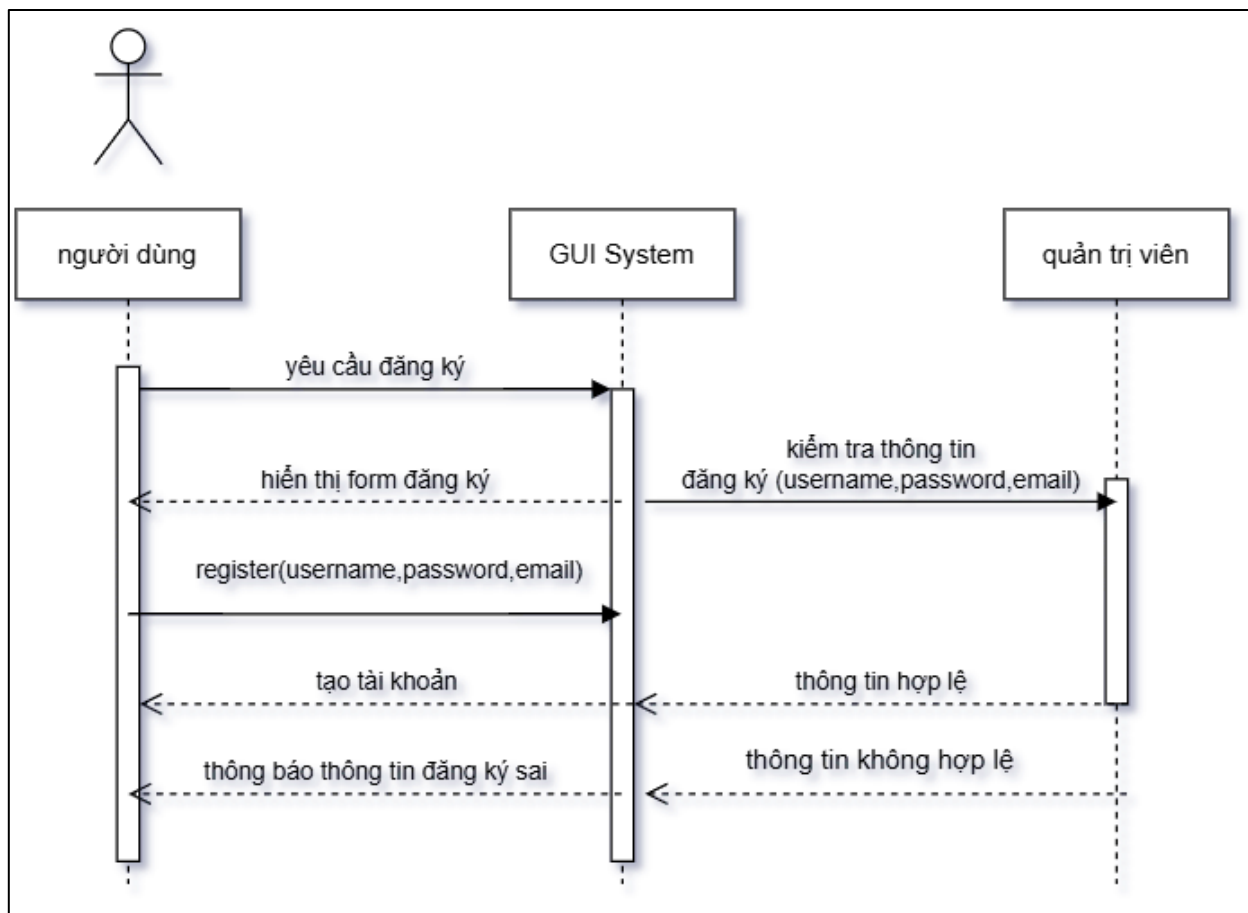
Hình 30.sơ đồ tuần tự-đăng ký
