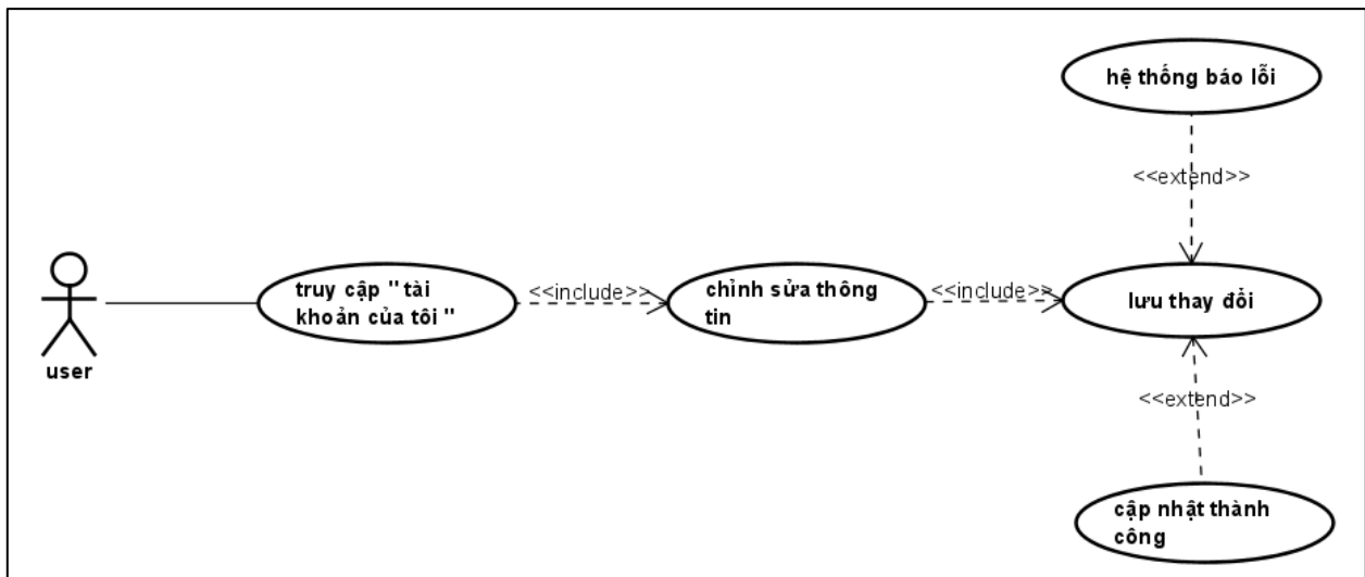
Hình 13.usecase quản lý tài khoản
