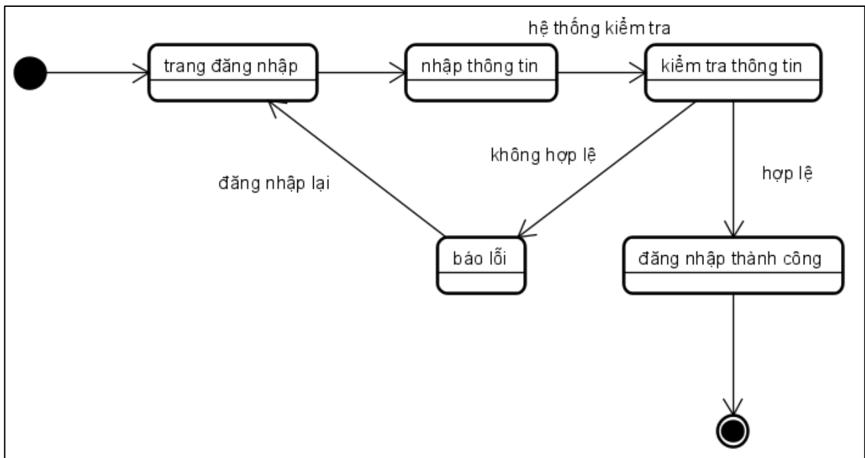
Hình 43.sơ đồ trạng thái-đăng nhập
