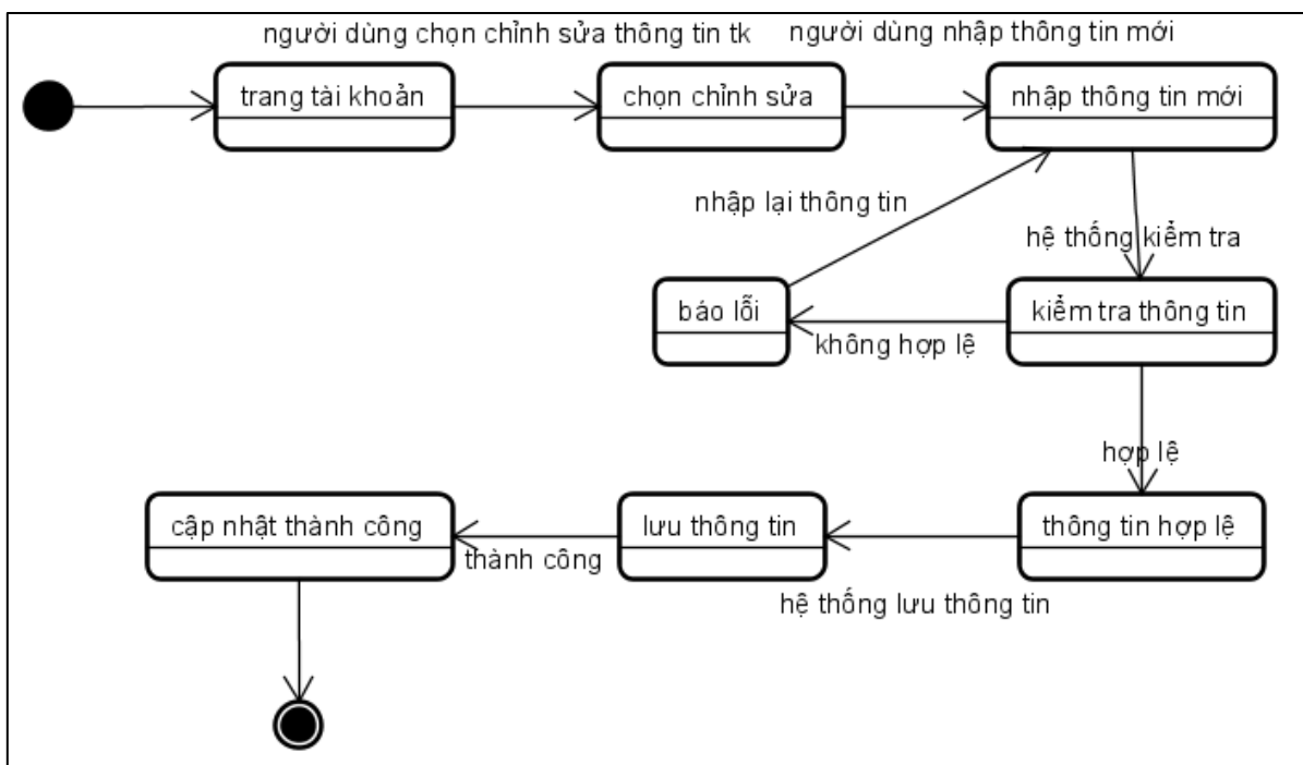
Hình 47.sơ đồ trạng thái-quản lý tài khoản
