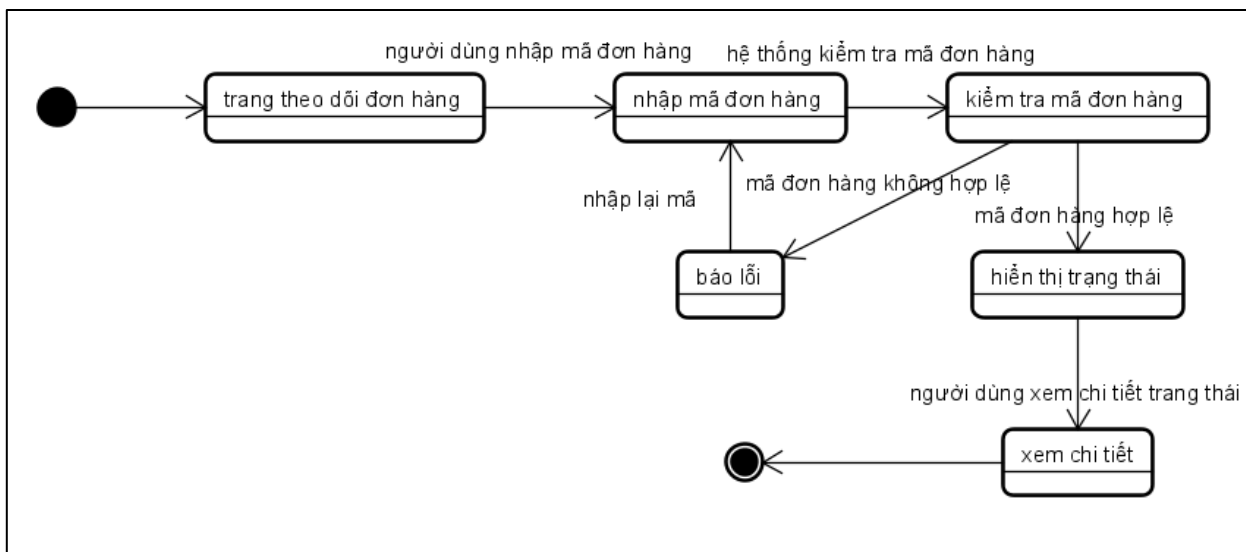
Hình 49.sơ đồ trạng thái-theo dõi đơn hàng
