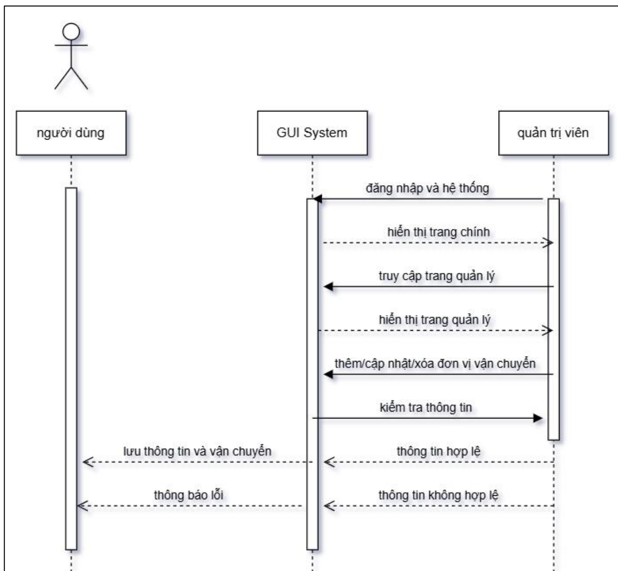
Hình 41.sơ đồ tuần tự-quản lý vận chuyển
