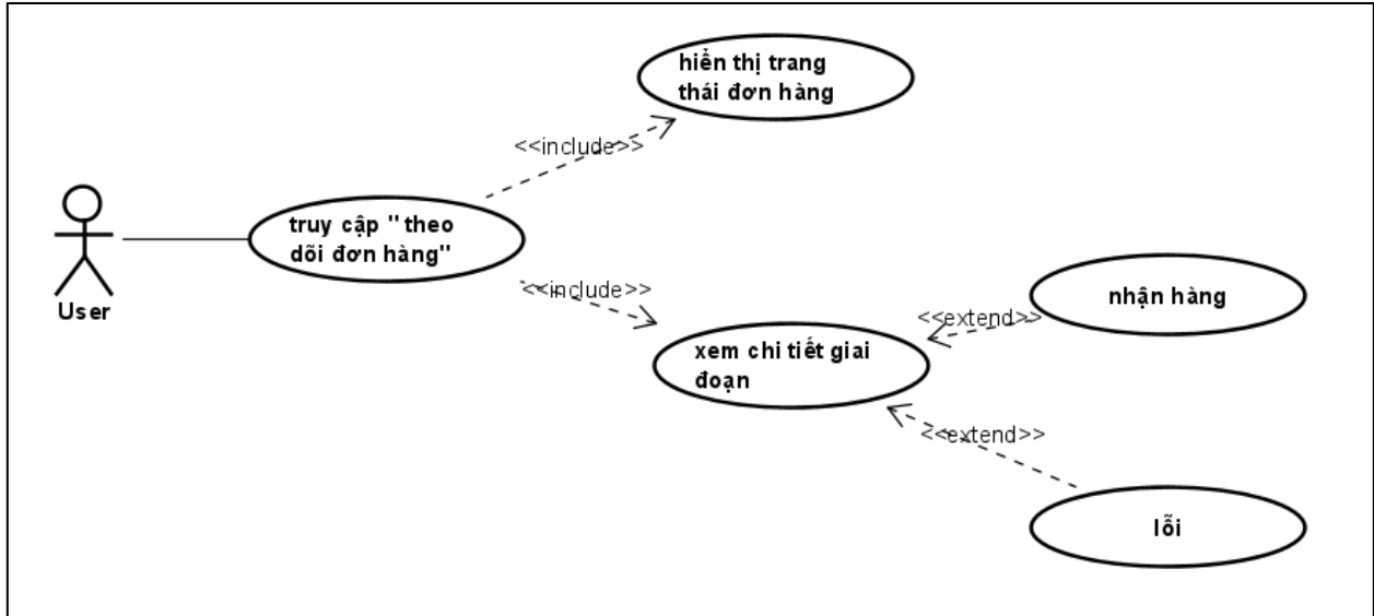
Hình 20.usecase theo dõi đơn hàng
