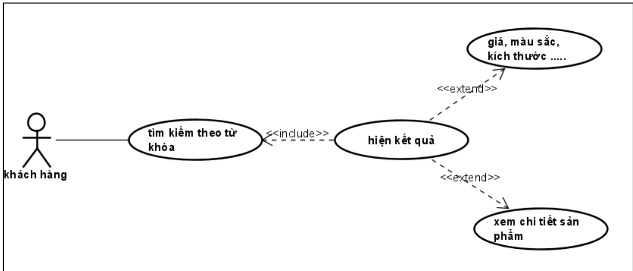
Hình 18.usecase tìm kiếm sản phẩm
