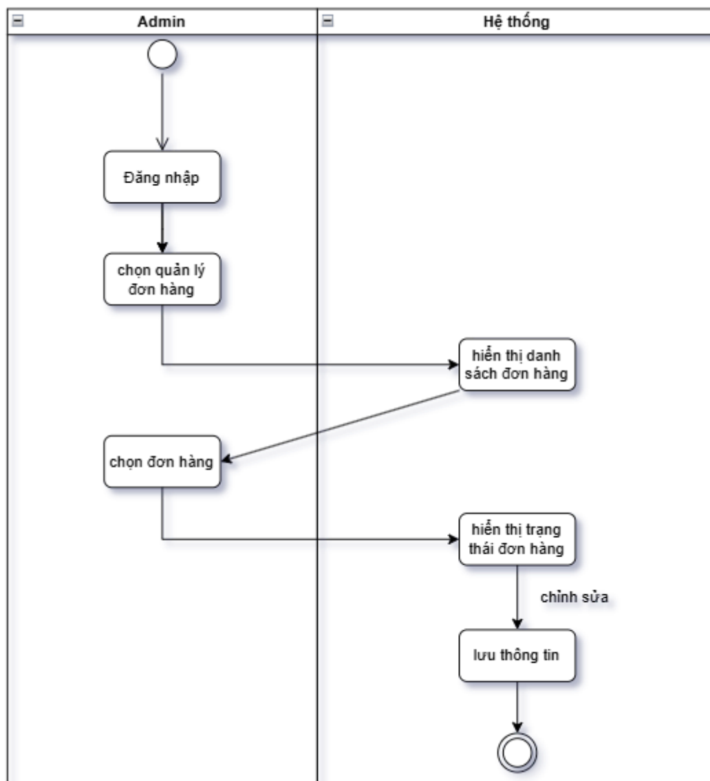
Hình 29.sơ đồ hoạt động-quản lý đơn hàng
