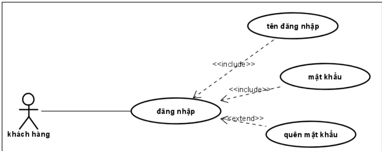
Hình 11. usecase đăng nhập
