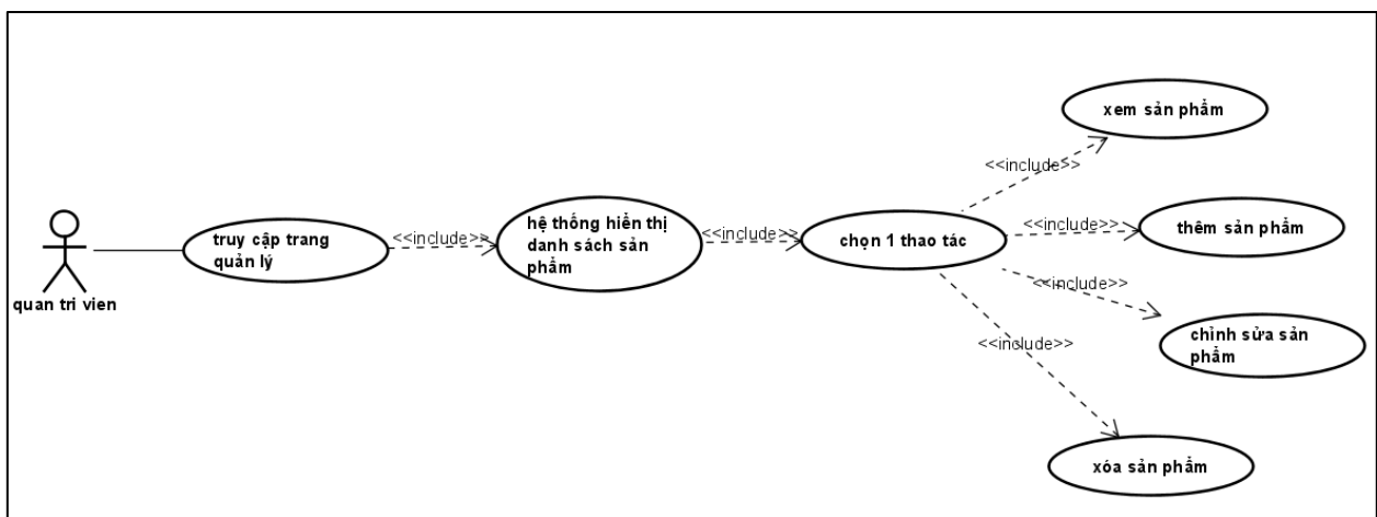
Hình 14. usecase quản lý sản phẩm
