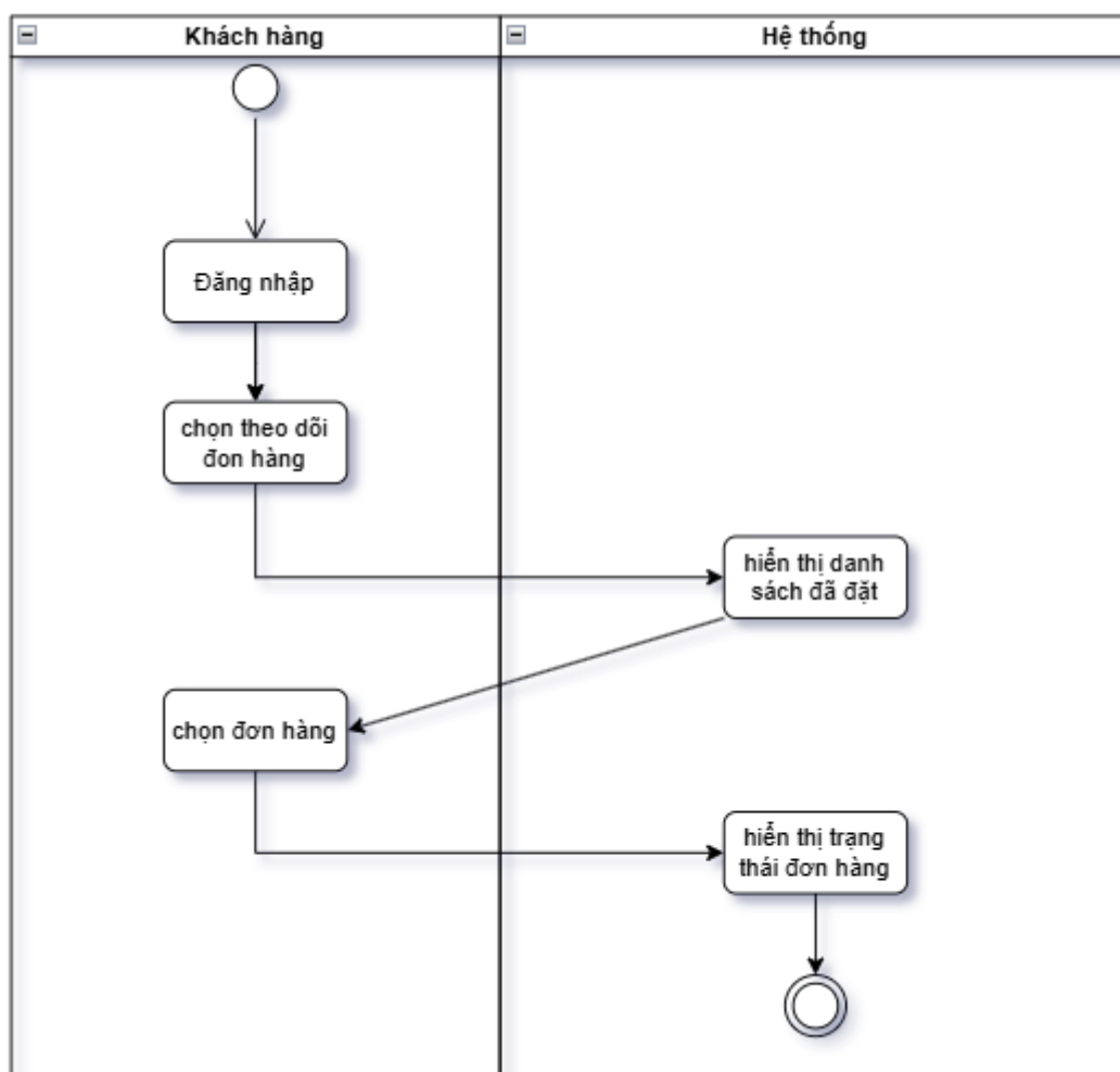
Hình 27.sơ đồ hoạt động-theo dõi đơn hàng
