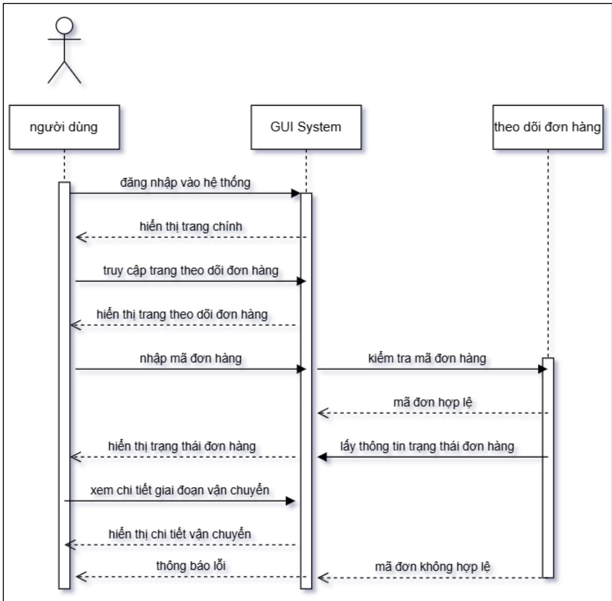
Hình 35.sơ đồ tuần tự-theo dõi đơn hàng
