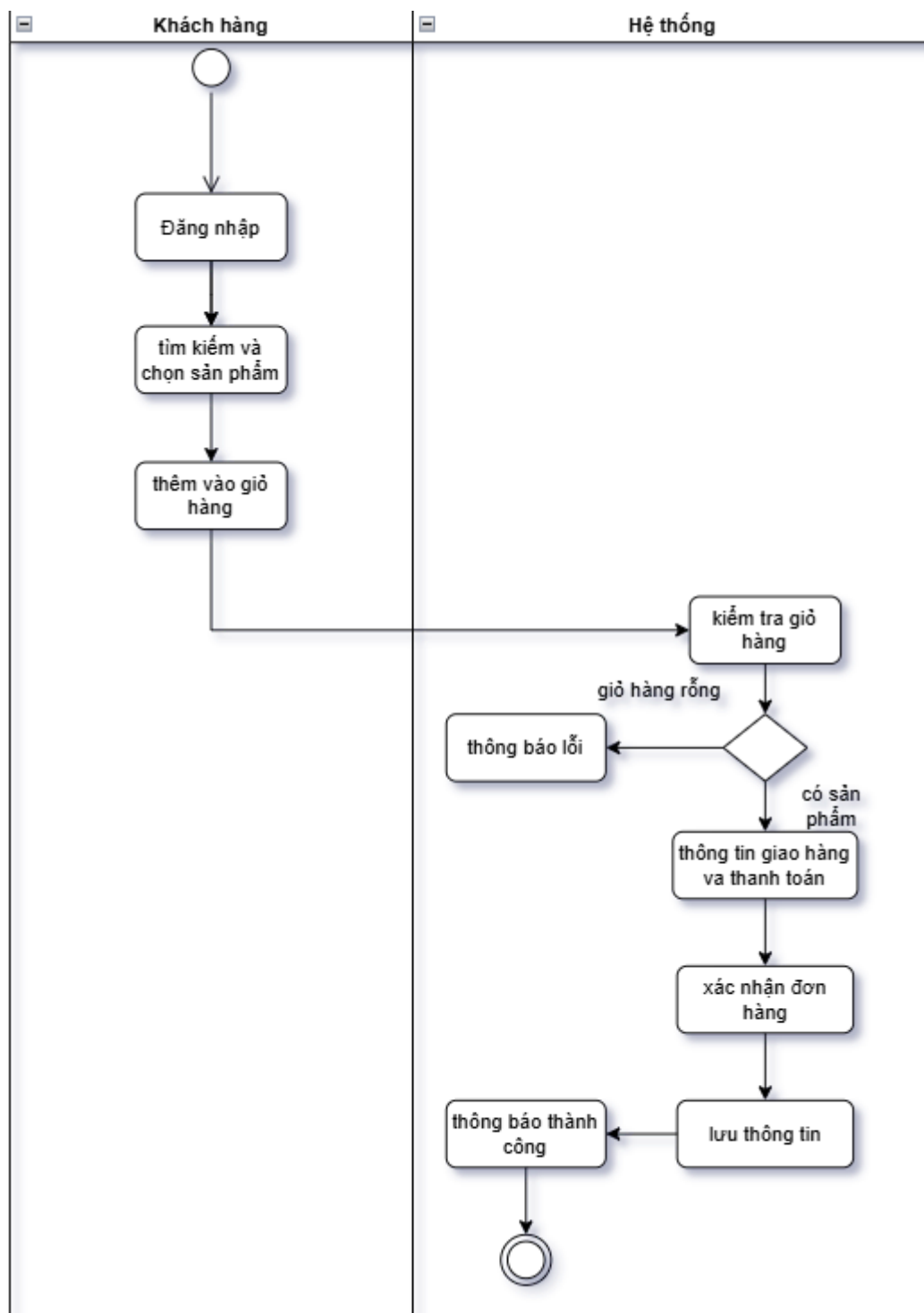
Hình 26.sơ đồ hoạt động-đặt hàng
