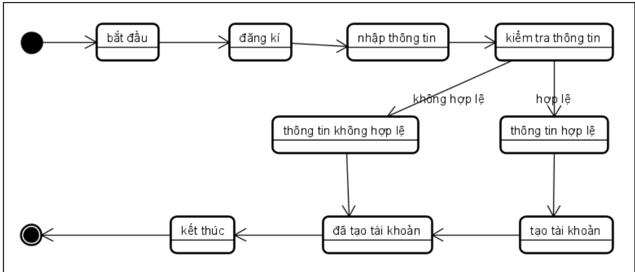
Hình 42.sơ đồ trạng thái-đăng ký
