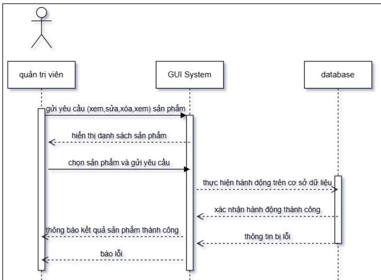
Hình 38.sơ đồ tuần tự-quản lý sản phẩm
