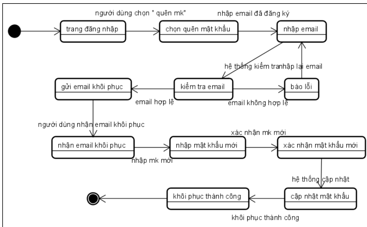
Hình 44.sơ đồ trạng thái-khôi phục mật khẩu
