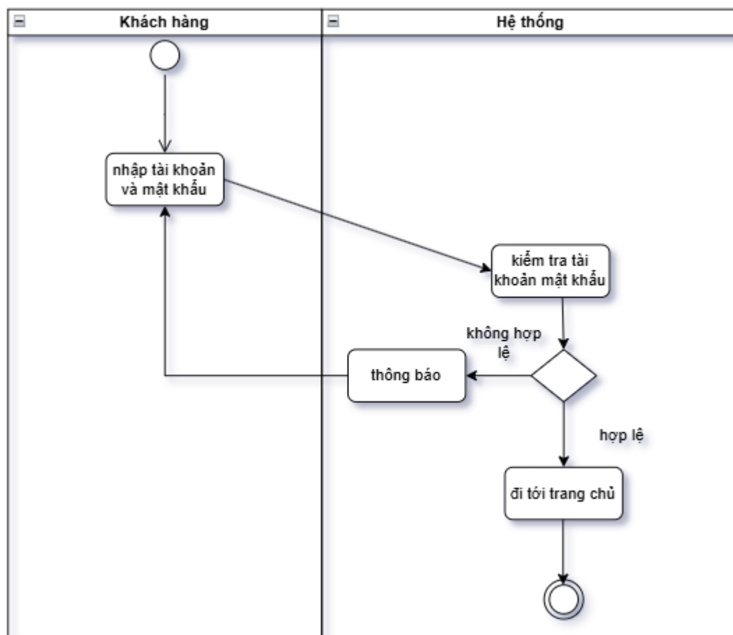
Hình 23.sơ đồ hoạt động-đăng nhập
