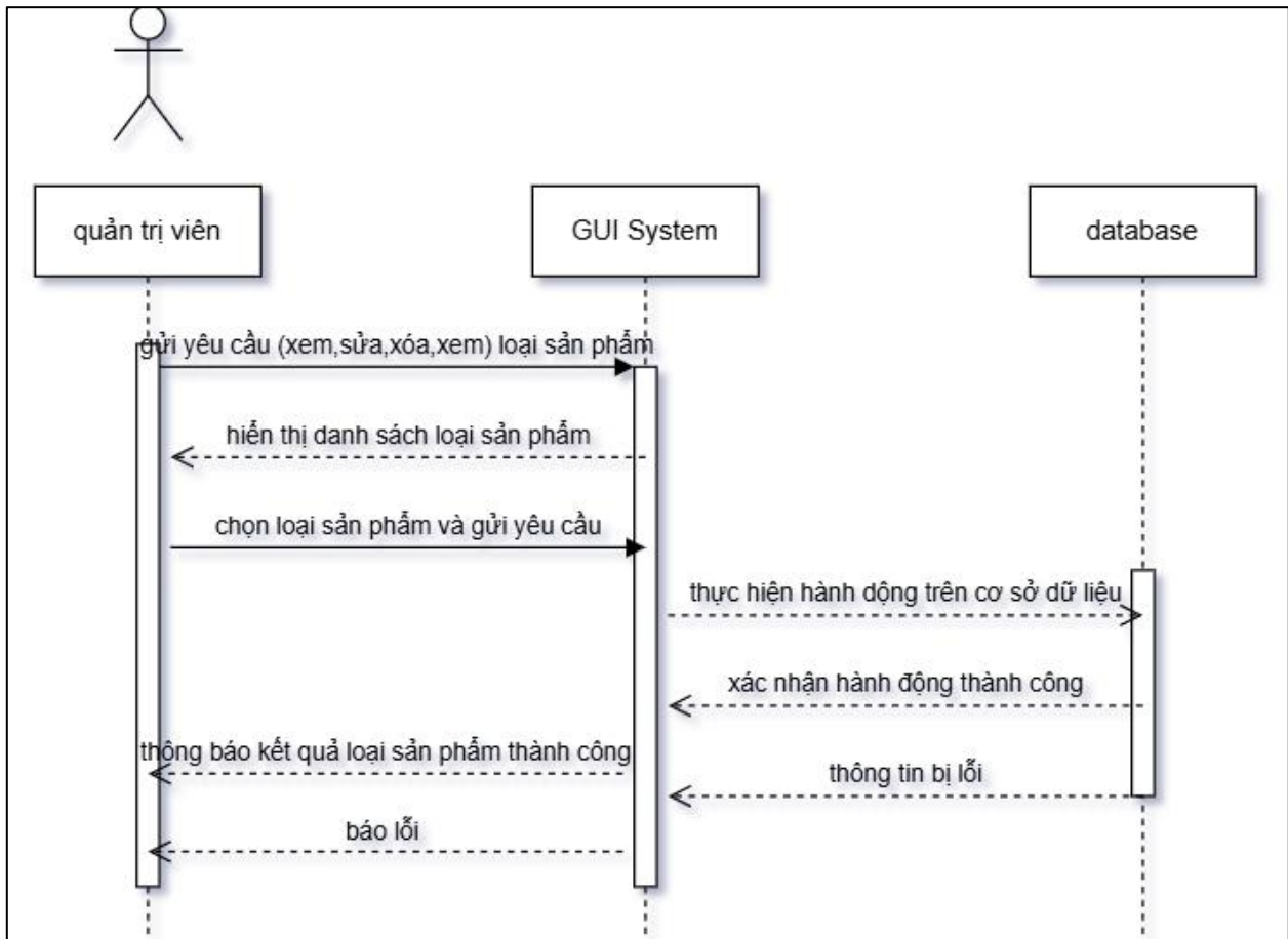
Hình 39.sơ đồ tuần tự-quản lý loại sản phẩm
