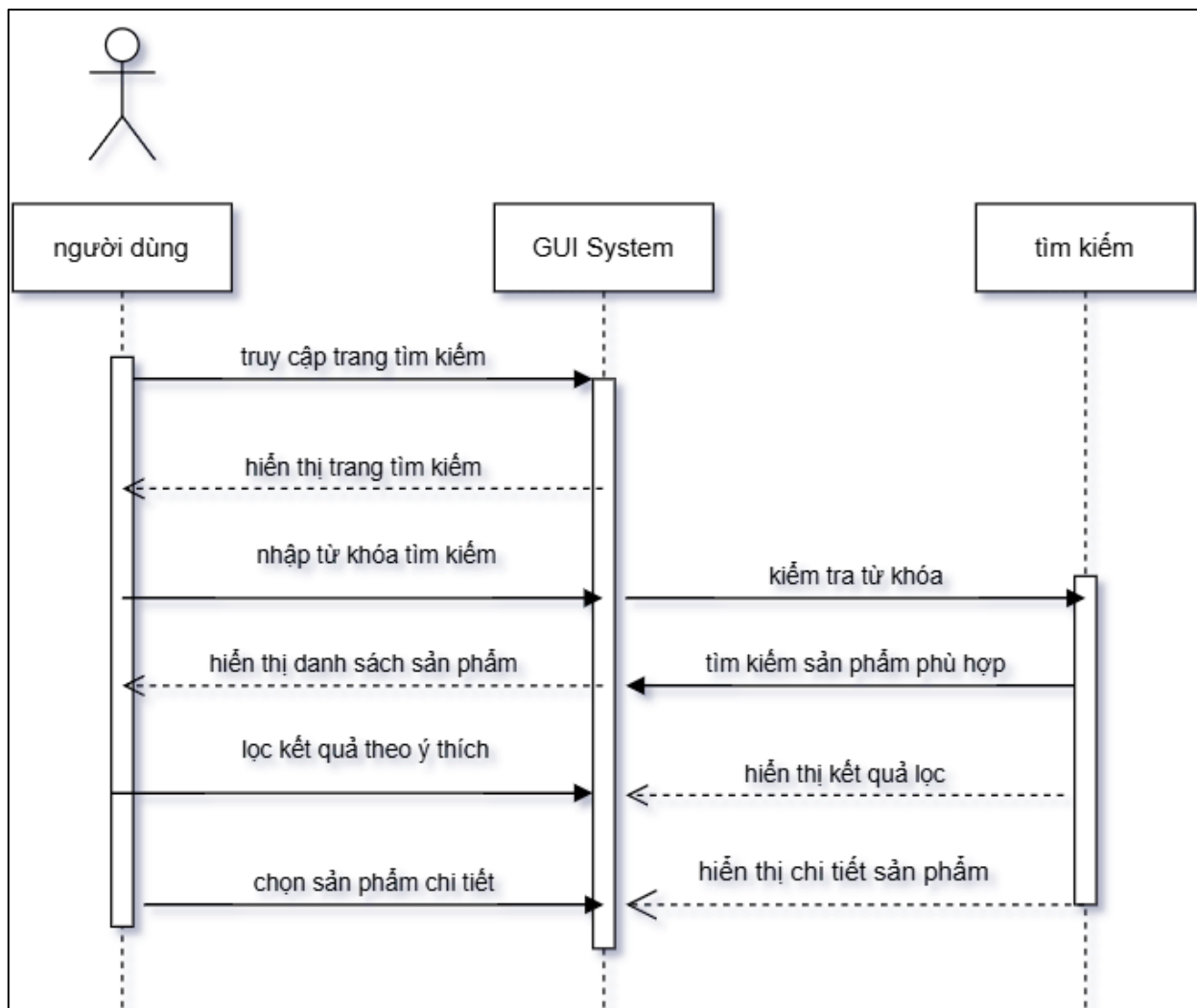
Hình 32.sơ đồ tuần tự-tìm kiếm
