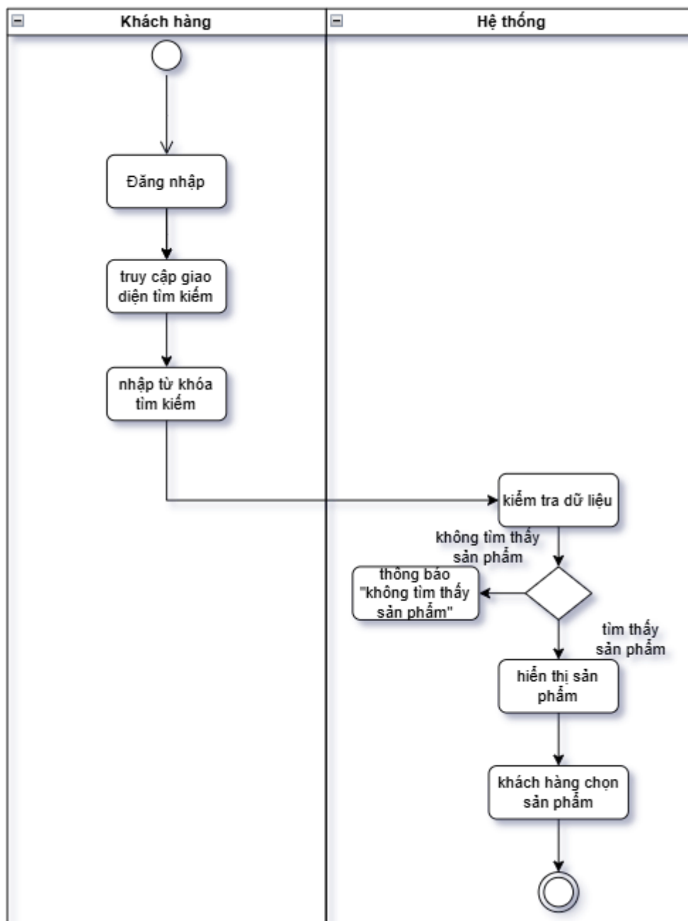
Hình 25.sơ đồ hoạt động-tìm kiếm
