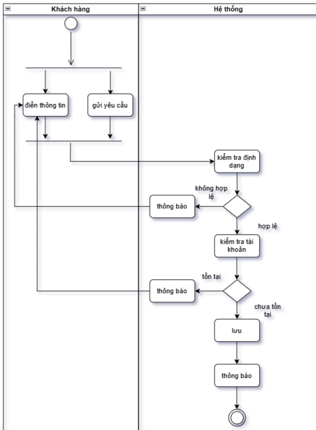
Hình 22.sơ đồ hoạt động-đăng ký
