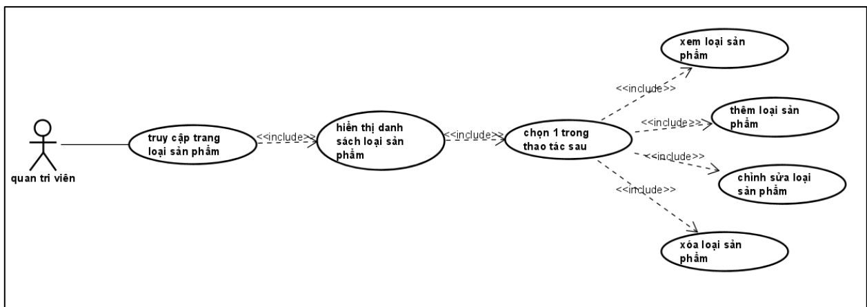
Hình 15.usecase quản lý loại sản phẩm
