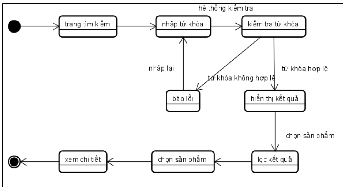
Hình 51.sơ đồ trạng thái-tìm kiếm
