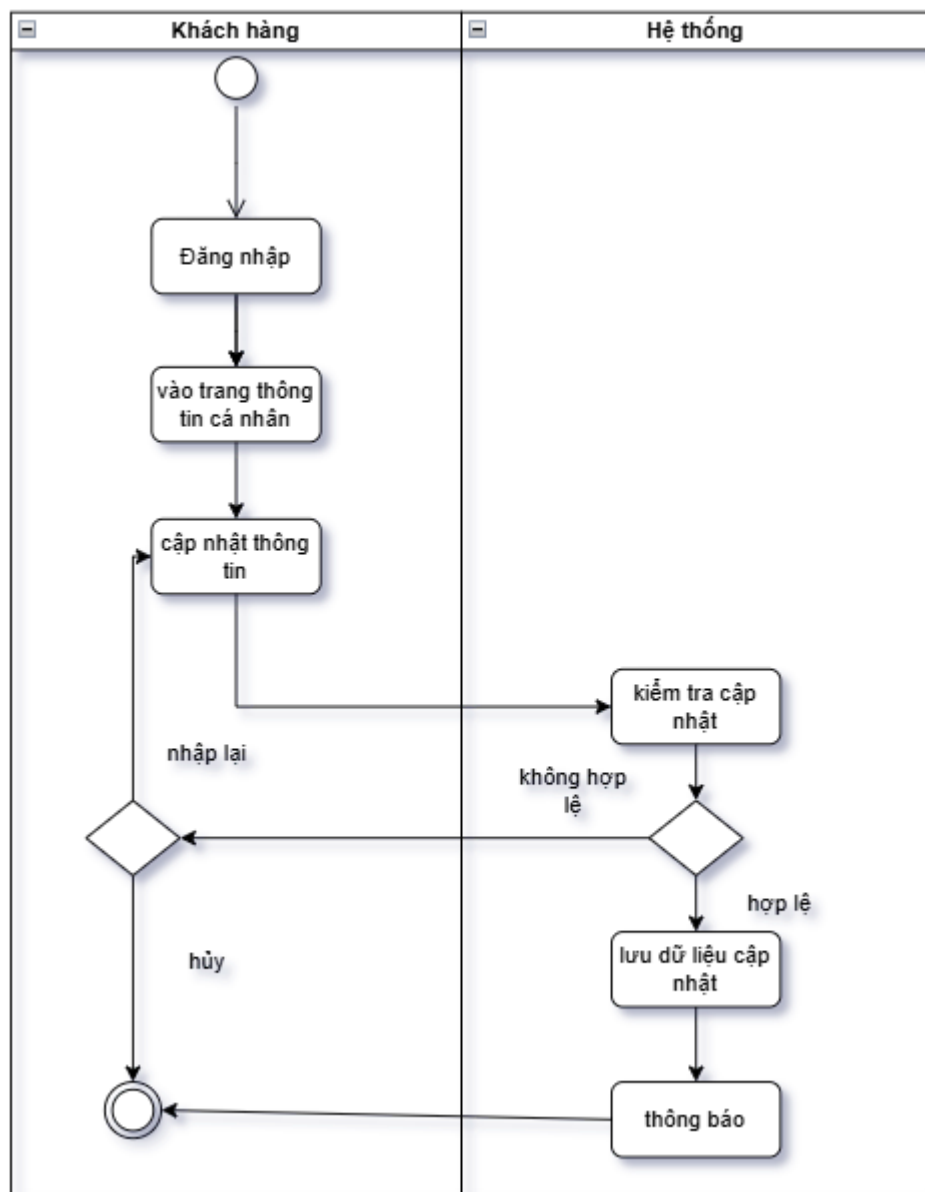
Hình 24.sơ đồ hoạt động-quản lý tài khoản
