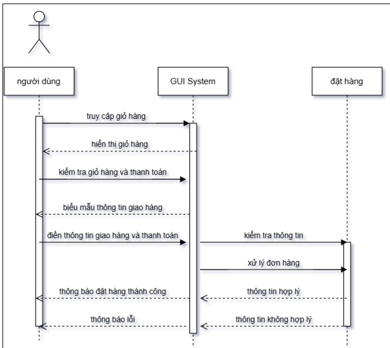
Hình 33.sơ đồ tuần tự-đặt hàng
