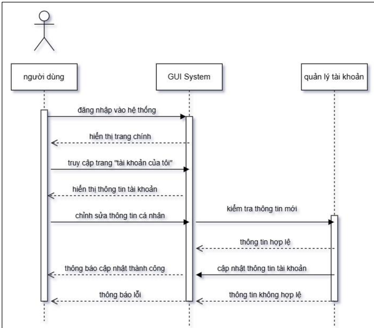
Hình 34.sơ đồ tuần tự-quản lý tài khoản
