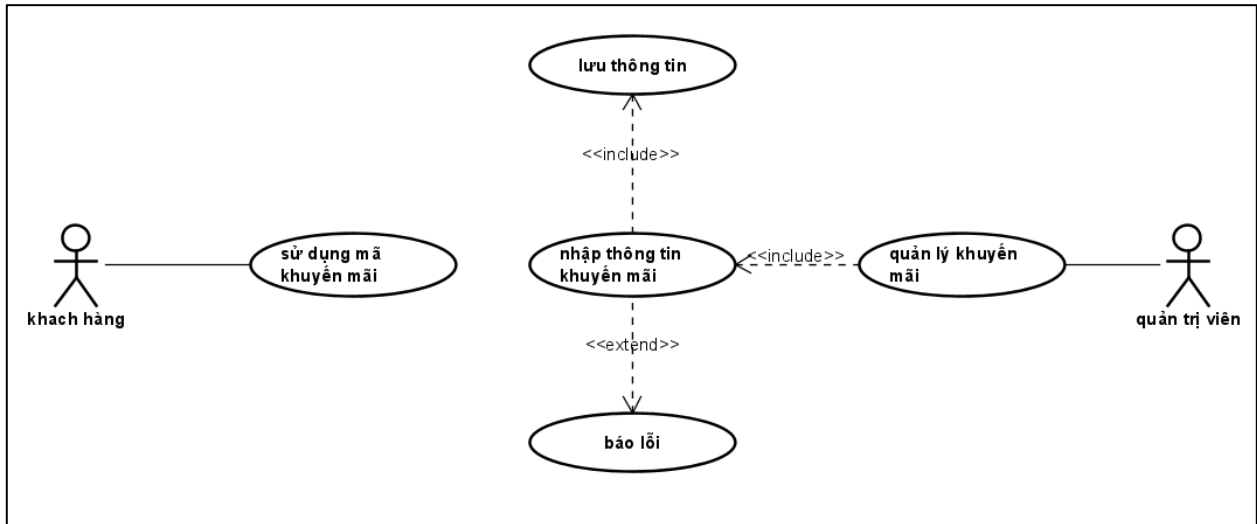
Hình 16. usecase quản lý khuyến mãi
