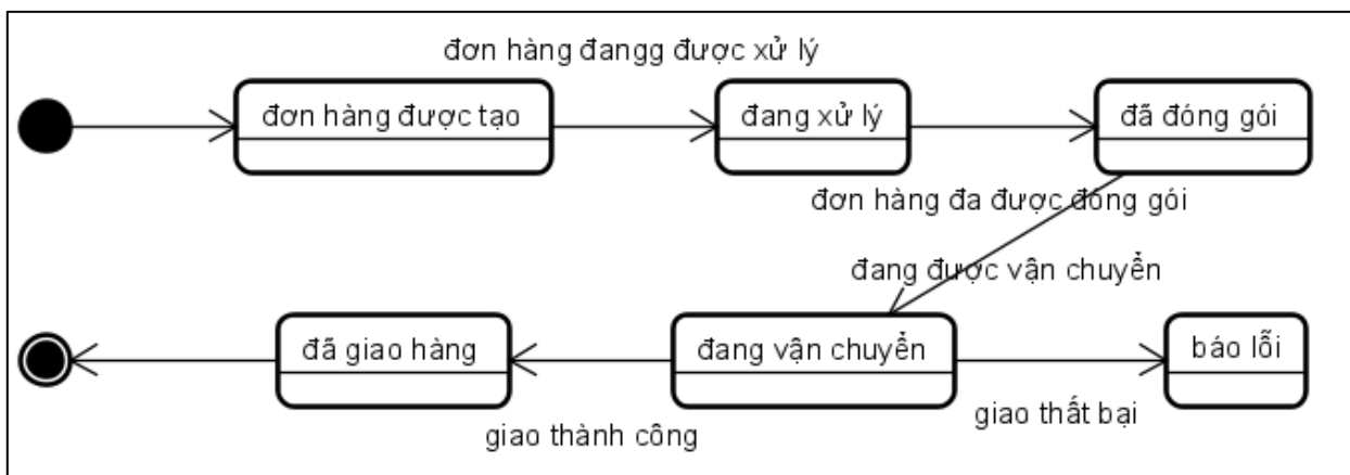
Hình 48.sơ đồ trạng thái-quản lý vận chuyển
