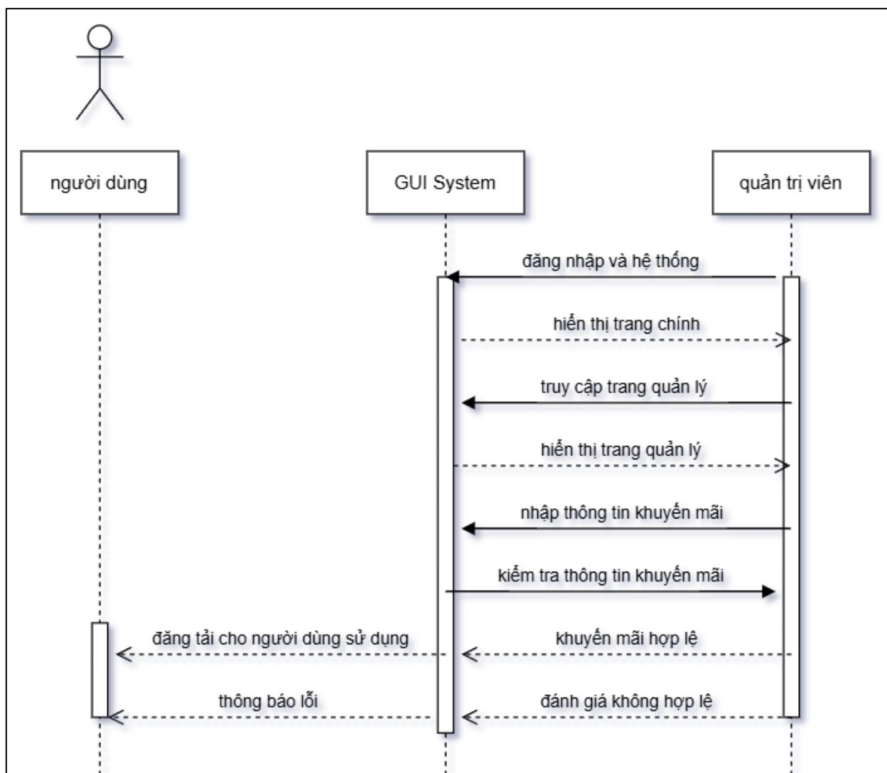
Hình 40.sơ đồ tuần tự-quản lý khuyến mãi
