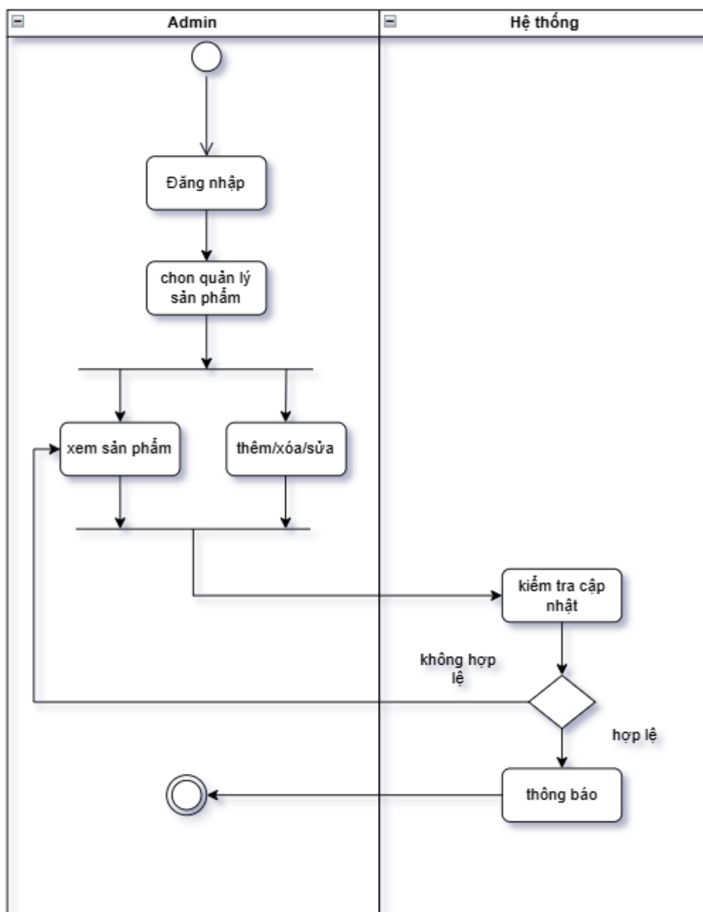
Hình 28.sơ đồ hoạt động-quản lý sản phẩm
