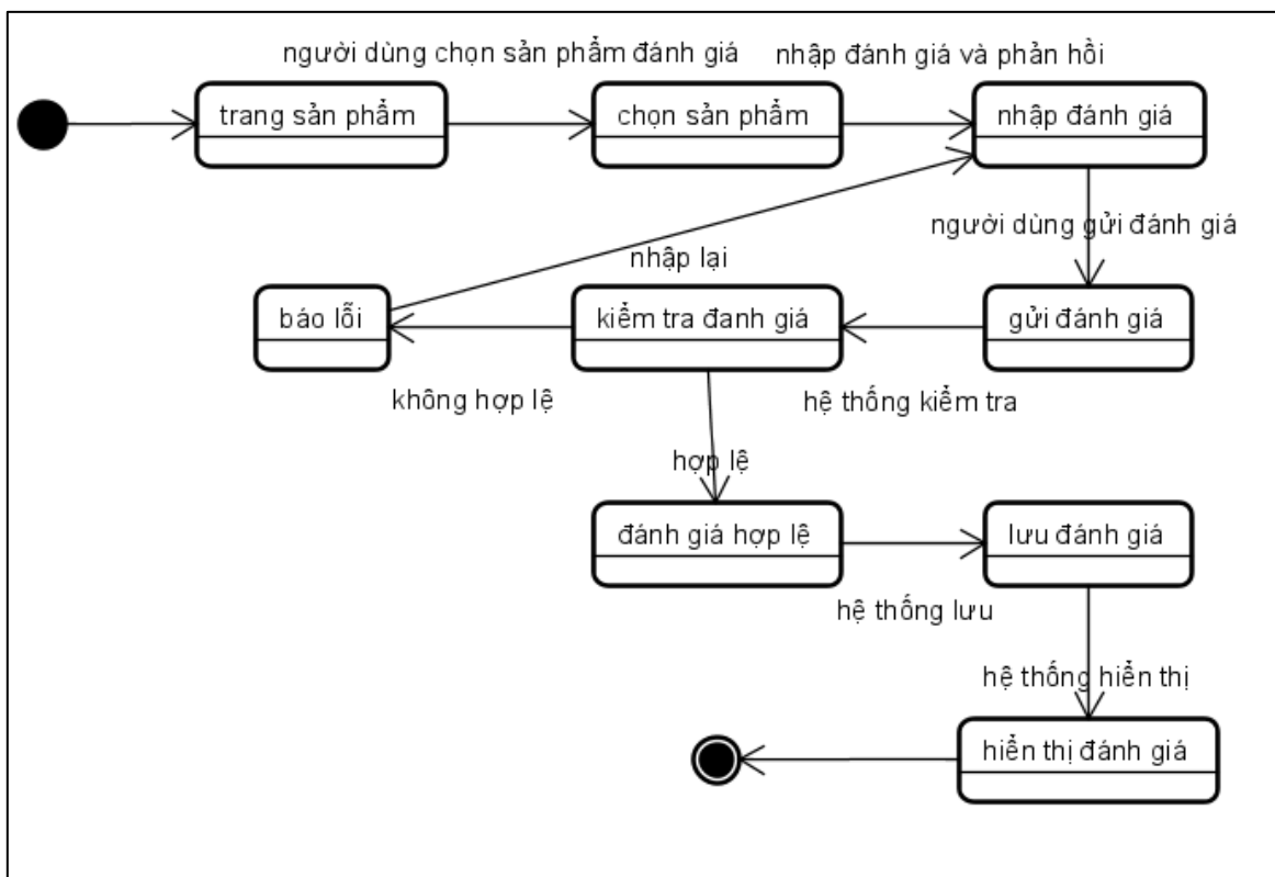
Hình 50.sơ đồ trạng thái-đánh giá phản hồi
