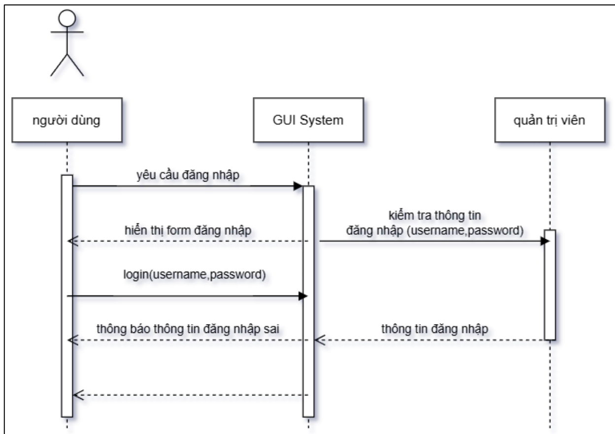
Hình 31.sơ đồ tuần tự-đăng nhập
