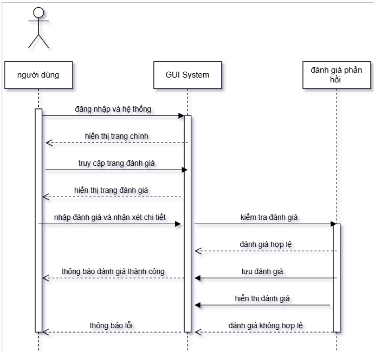
Hình 37.sơ đồ tuần tự-đánh giá phản hồi
