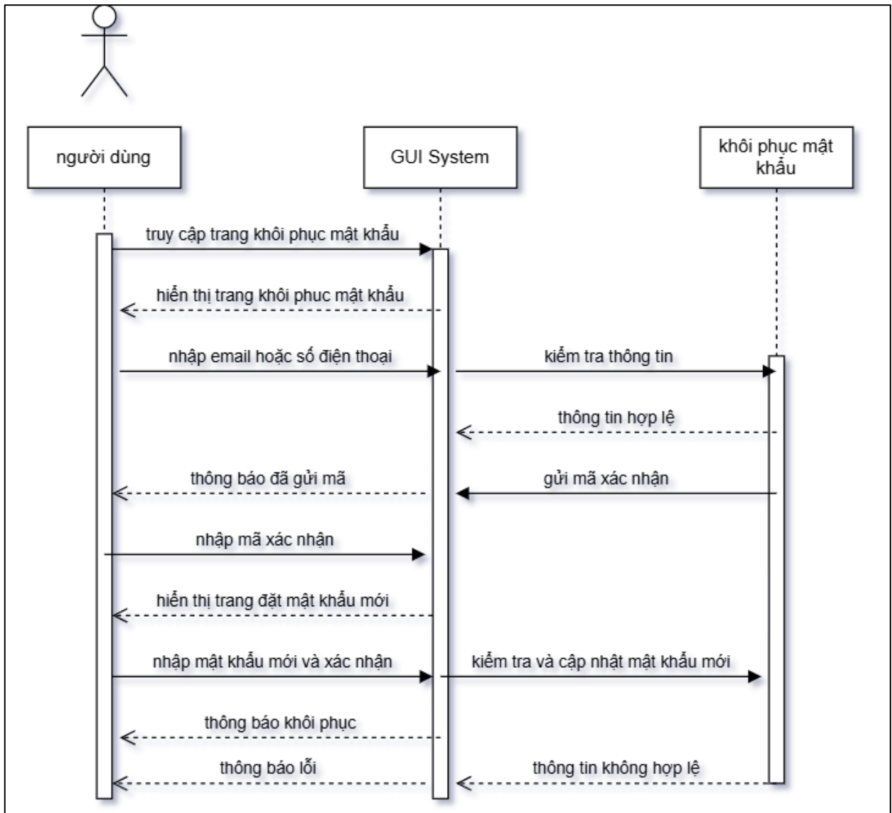
Hình 36.sơ đồ tuần tự-khôi phục mật khẩu
