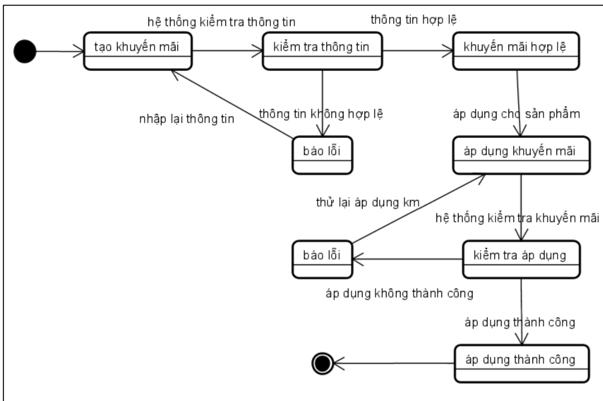
Hình 46.sơ đồ trạng thái-quản lý khuyến mãi
