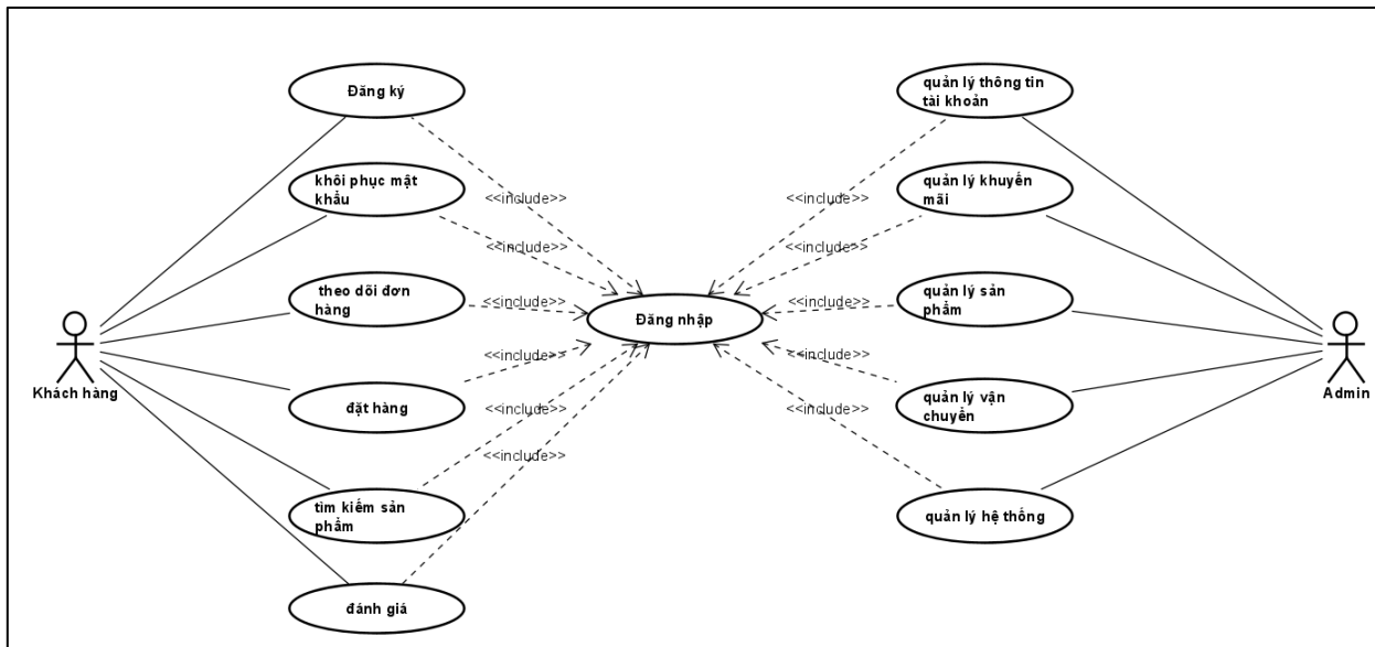
Hình 9.usecase phân rã chức năng
